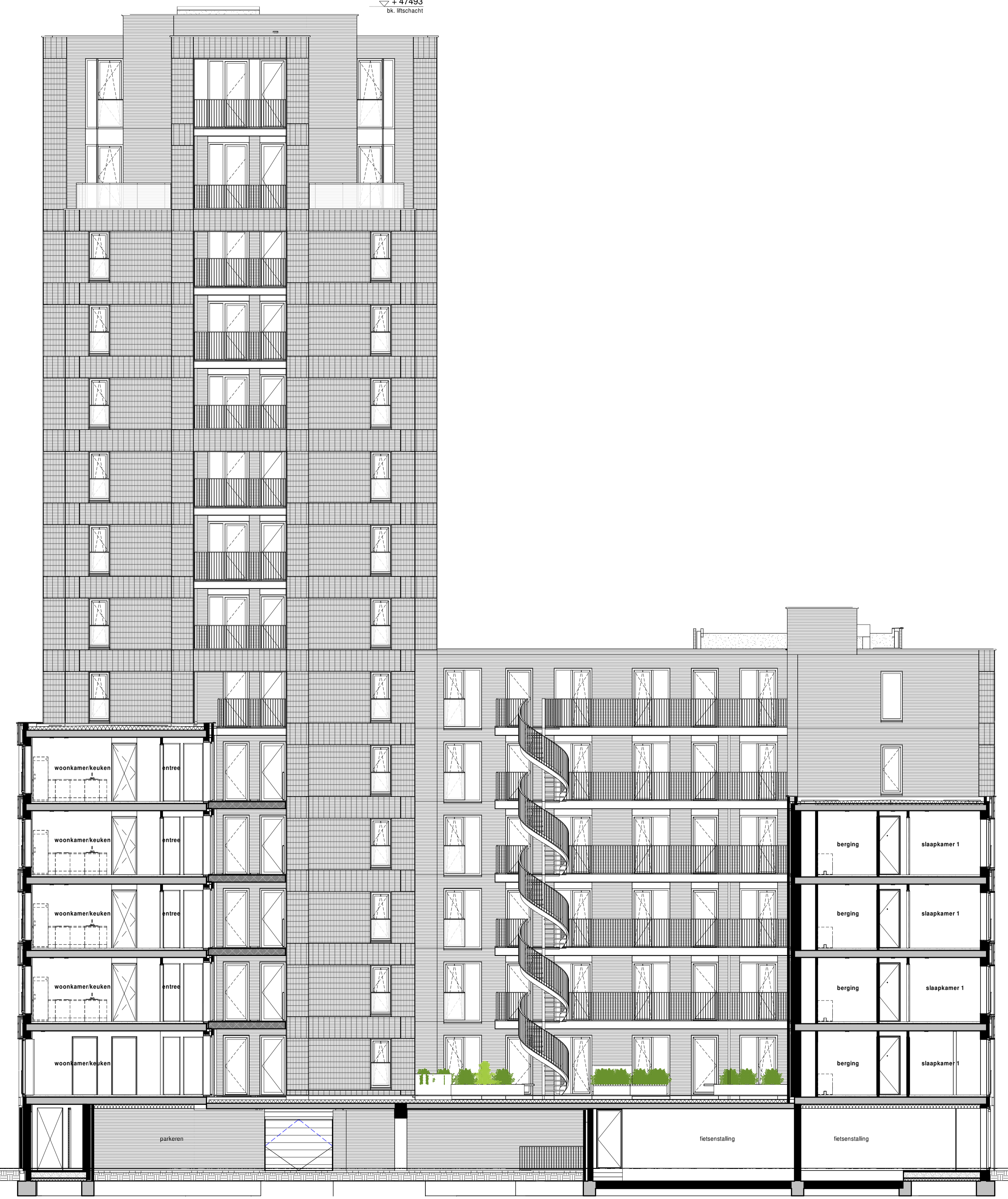
Doorsnede B-B
